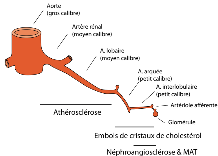
Figure 1. Arbre vasculaire
